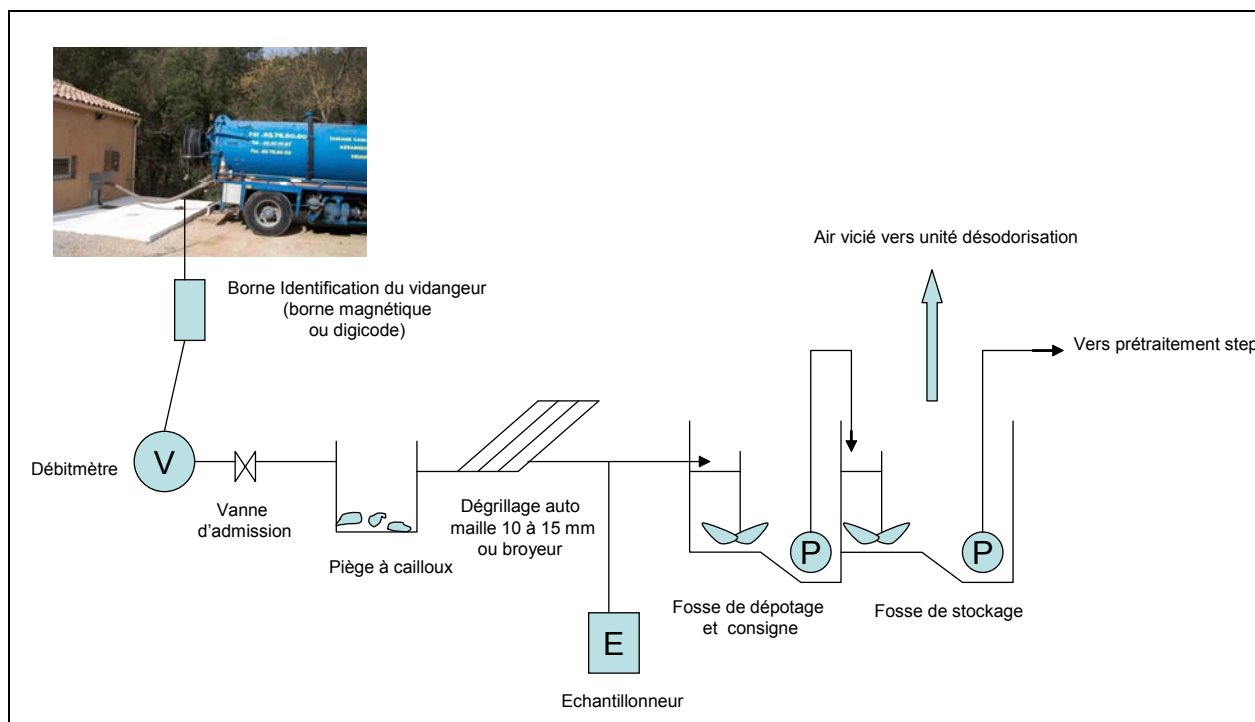
Figure 9 : Schéma simplifié d'une unité de réception des matières de vidange
