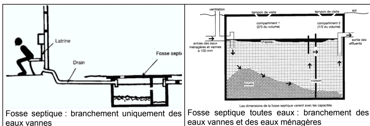
Figure 1 : différentes fosses (source guide de l'assainissement individuel, OMS, 1995)
