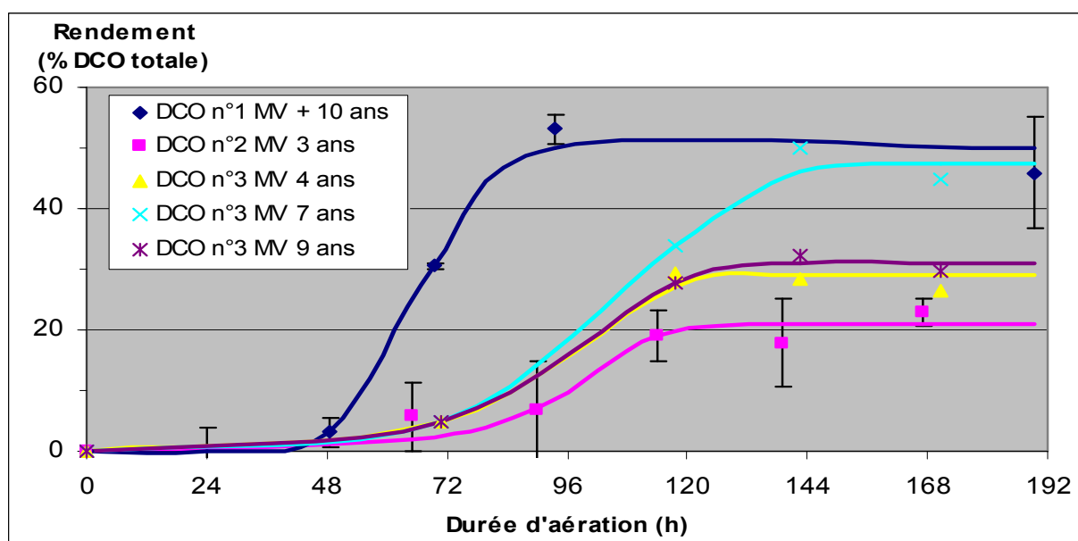
Figure 8 : Rendement épuratoire sur la DCO totale de chaque matière de vidange, lors de leur aération.
