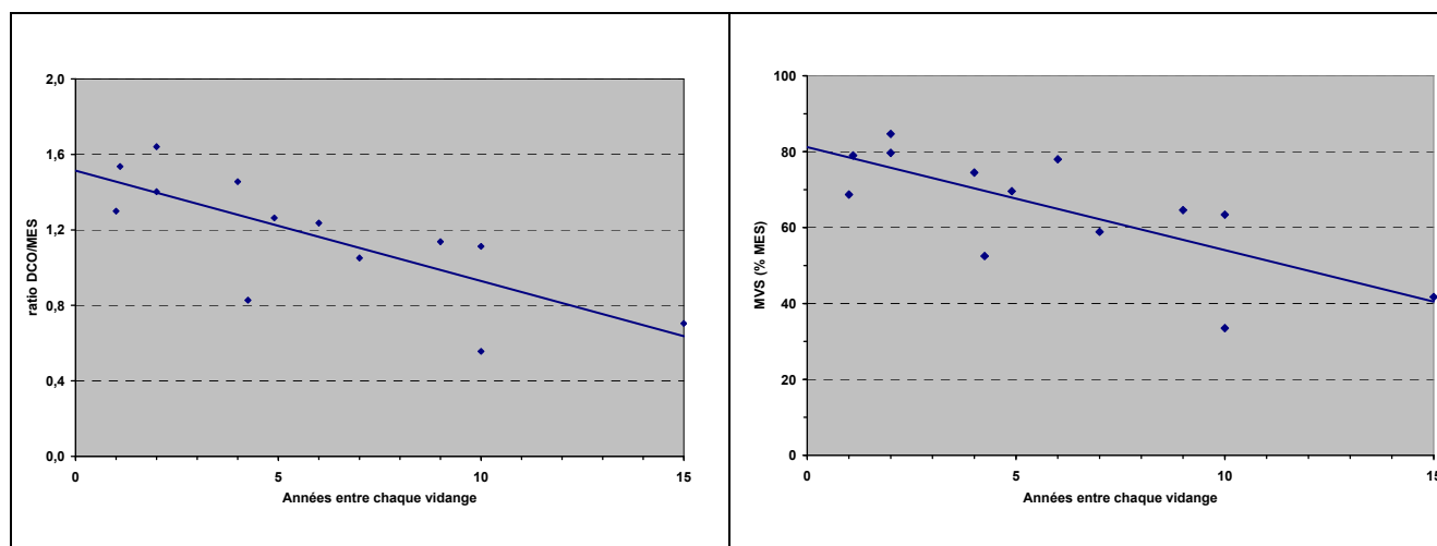
Figures 4 et 5 : exemples d'augmentation du ratio DCO/DBO 5 dans le temps, et de diminution du ratio DCO/MES dans le temps, s'accompagnant d'une baisse du taux de MVS.
